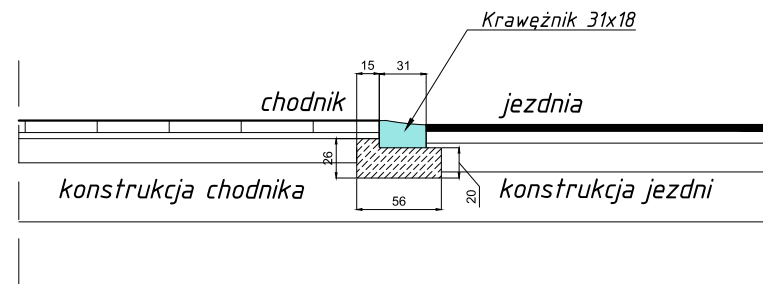
Przekrój poprzeczny elementu w miejscu przejścia niepełnosprawnego na wózku
