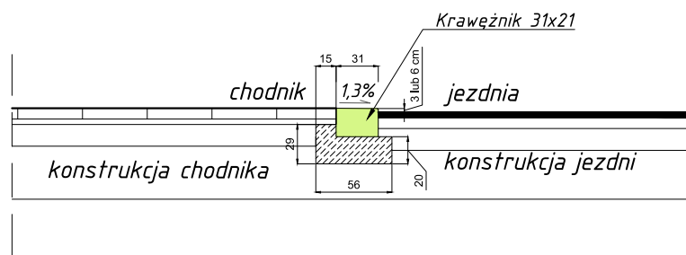
Przekrój poprzeczny elementu w miejscu przejścia niewidomego
